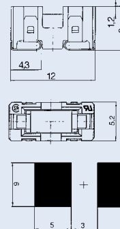
Solder pads / Anschlussflächen
