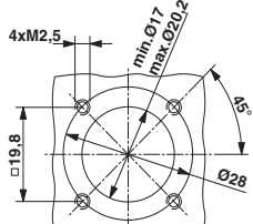
Einbaumaße: ST-17.1N8AAC00S
