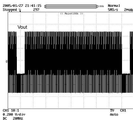
Fig.31 Vout (C=1000µF)
