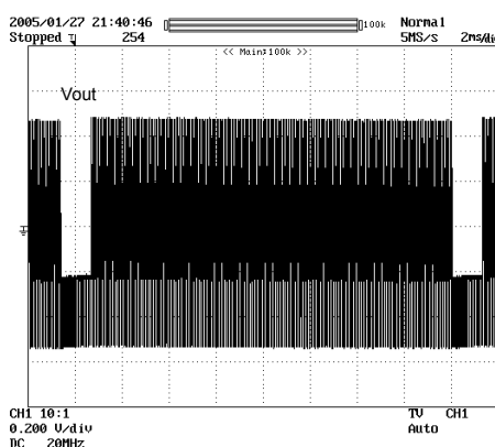
Fig.30 Vout (C=220µF)
