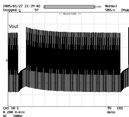
Fig.29 Vout (C=22µF)
