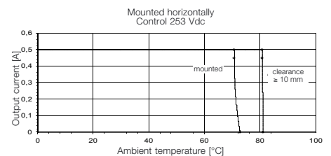
WOS 1 230 VUC • 8275380000
