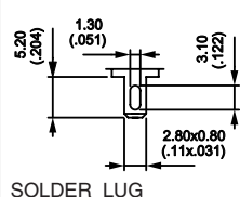
SOLDER LUG
