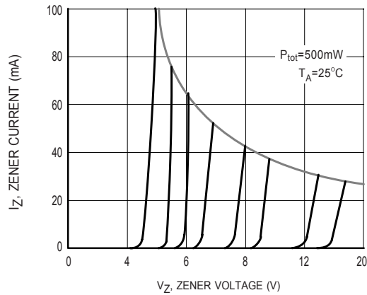
Figure7 Zener Current vs. Zener Voltage
