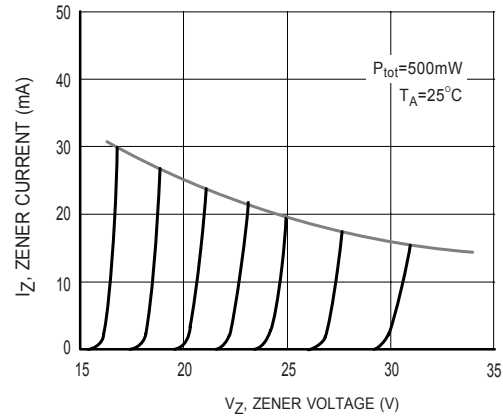
Figure8 Zener Current vs. Zener Voltage
