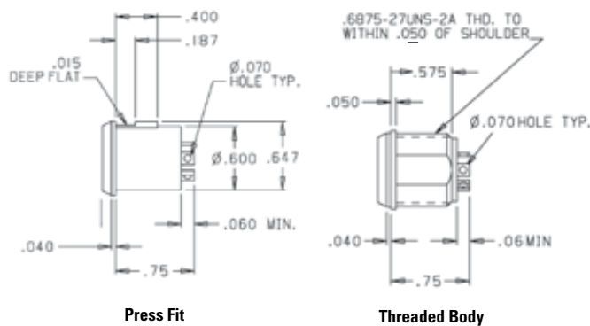
Press Fit
