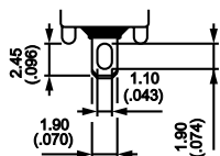
Solder lug terminal
