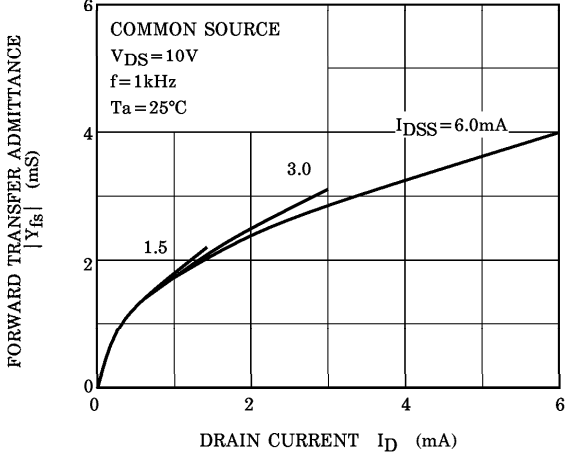
|Y_{fs}| - I_D
