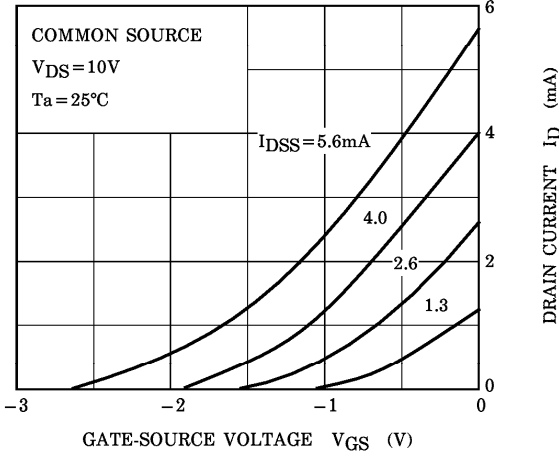
I_D - V_{GS}
