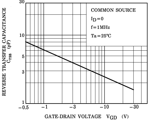
C_{rss} - V_{GD}
