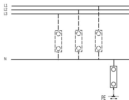
TT network (PUD 100 Neutre)
