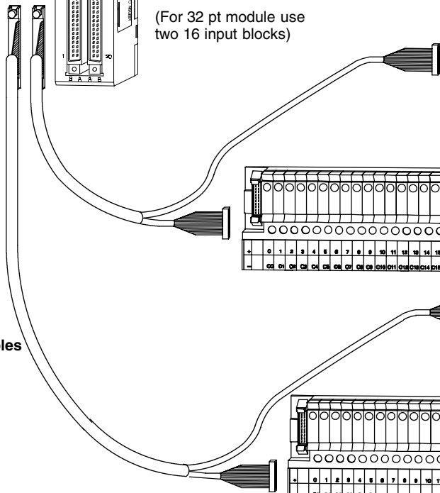
Input Module C200H-ID216 C200H-ID217
