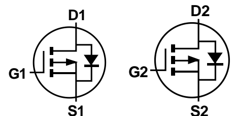
Q1 P-CHANNEL
