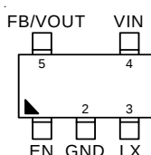
SOT-23-5/TSOT-23-5
