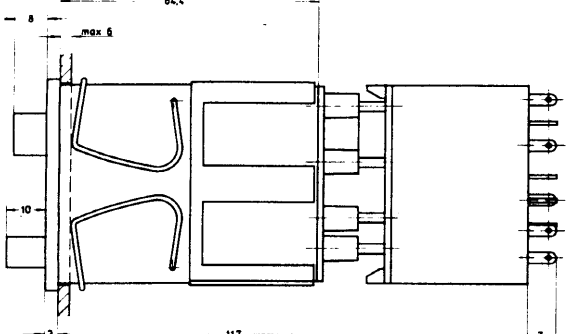
FR 329 Cutout 50,5 x 50,5 mm
