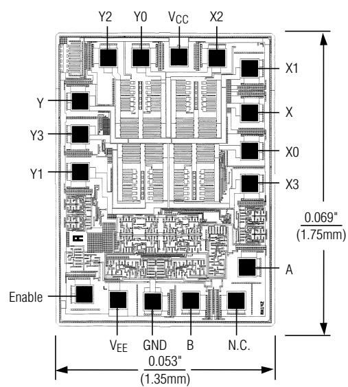
MAX4582
