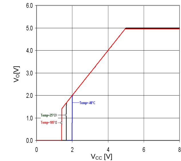
Figure 27. Vcc-Vo (Io=0mA)
