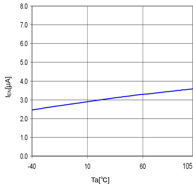
Figure 24. Ta-I EN
