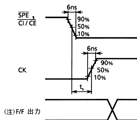
波形 5
