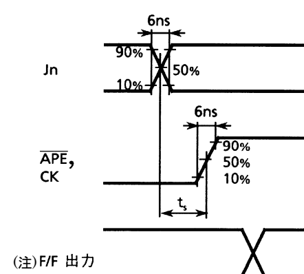
波形 6
