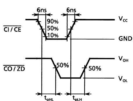
波形 4
