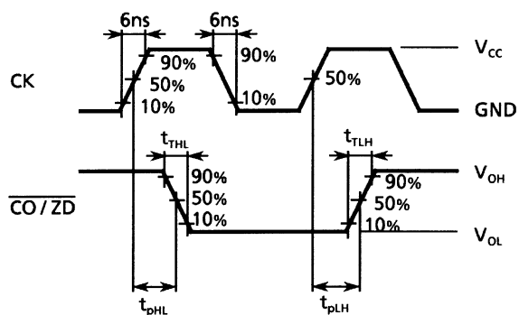
波形 1
