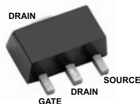
TO-243AA (SOT-89) (N8)
