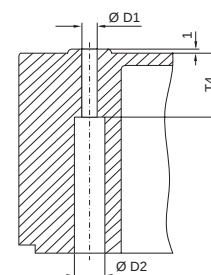
Schnitt A – A
