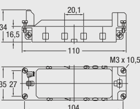
Montageausschnitt/Panel cut-out
