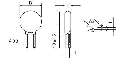
(ERZV10D182CS)
