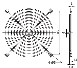
FG-12 For 120mm Fan
