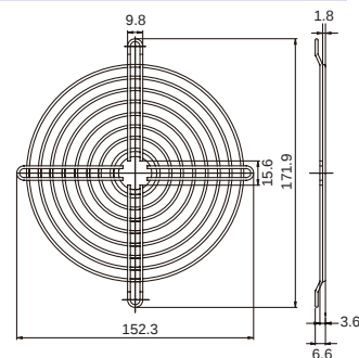
FG-17A For 172mm Fan
