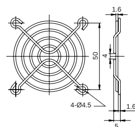
FG-06 For 60mm Fan
