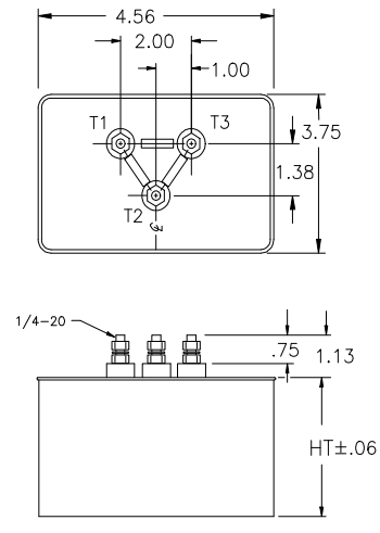
FIG. 2 (SUFFIX "33S")
