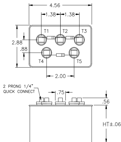
FIG. 1 (SUFFIX "35")
