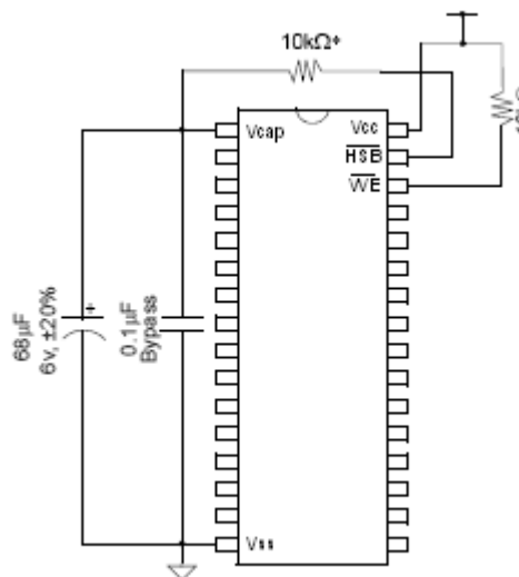
Figure 2. AutoStore Mode
