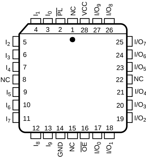
PLCC JEDEC
