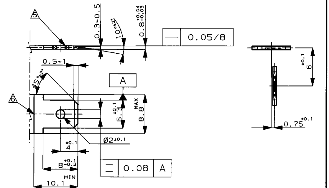
タブ寸法推奨図 RECOMMENDED MATING TAB DESIGN
