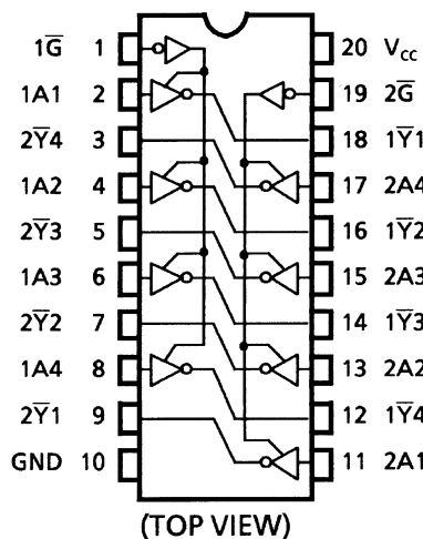
TC74HC240A
