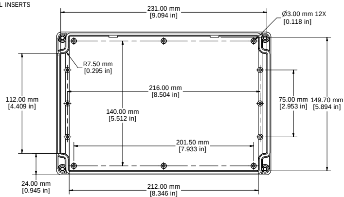
LID - INSIDE
