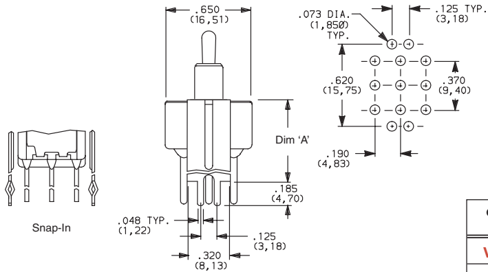
7301MD9__BE 3PDT
