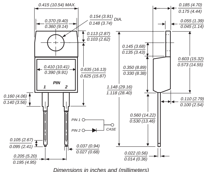
TO-220AC
