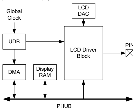
图 8-6. LCD 系统
