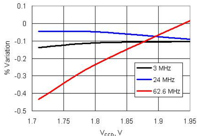
图 11-61. IMO 频率变化与 V CC
