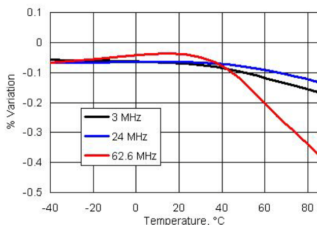
图 11-60. IMO 频率变化与温度
