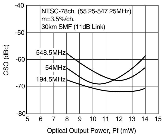
Fig. 10 CSO vs. Output Power
