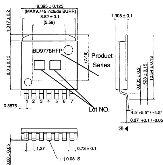
HRP7 (UNIT:mm)
