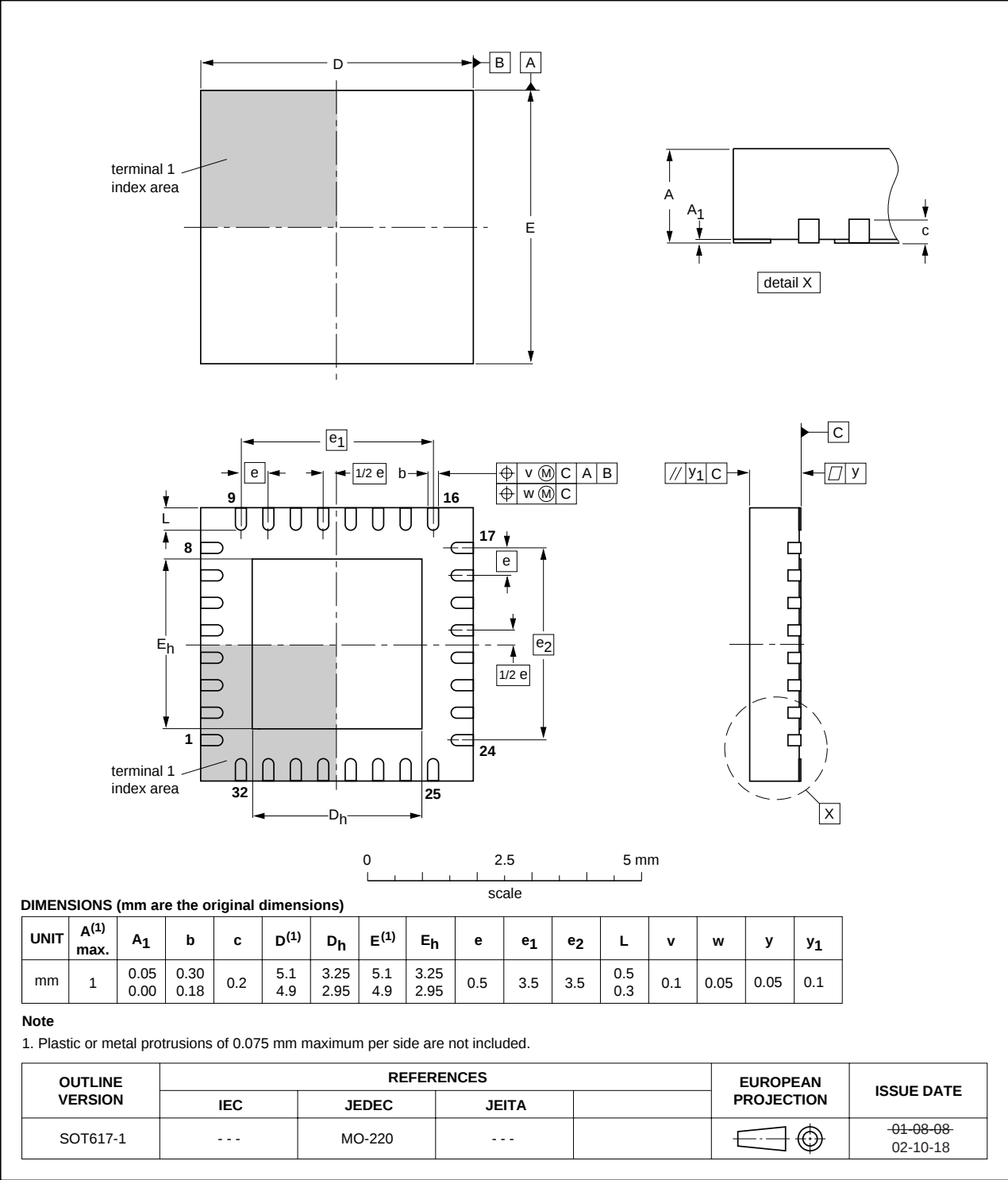
Fig 19. Package outline SOT617-1
