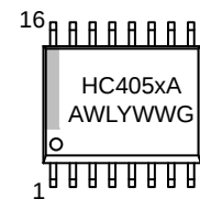
SOIC-16 WIDE
