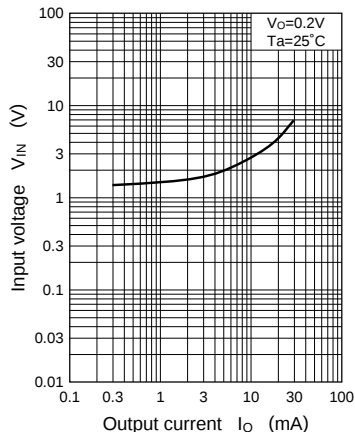
V_{IN} - I_O
