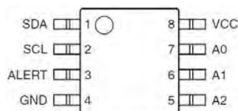
SOIC (3.9 x 4.9 mm)
