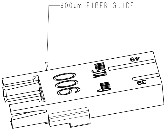
900um FIBER GUIDE
