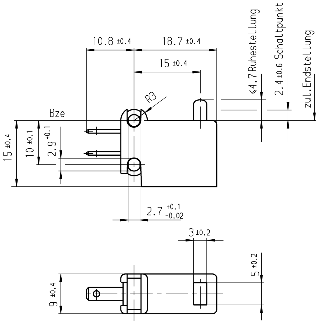
Flachstecker DIN 46 244-A 2,8-0,8 (EN 61058 / EN 61210)
