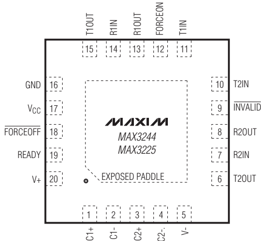
TQFN
