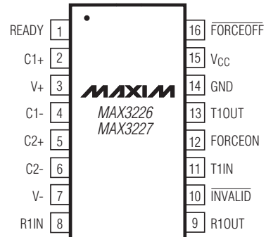
SSOP
