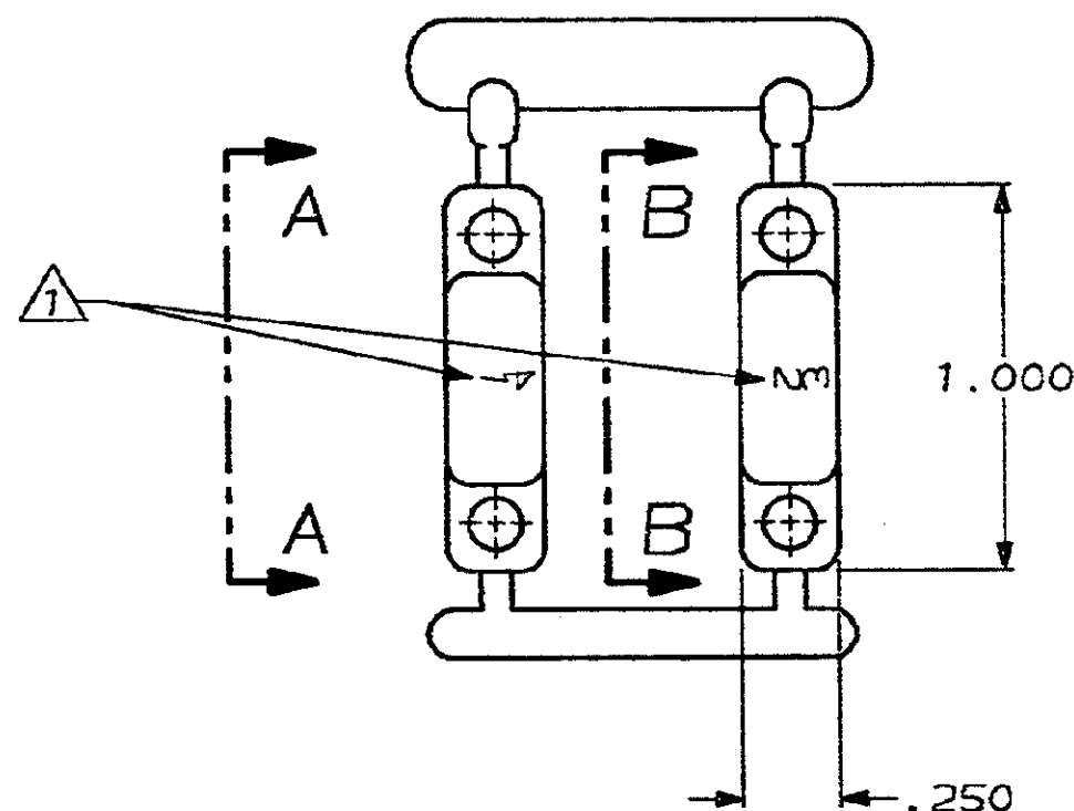
VIEW A-A
