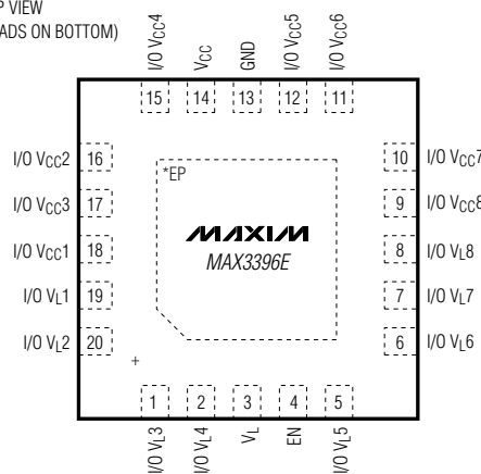
TQFN
