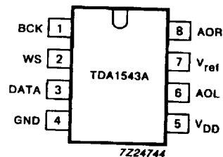
Fig.2 Pinning diagram.
