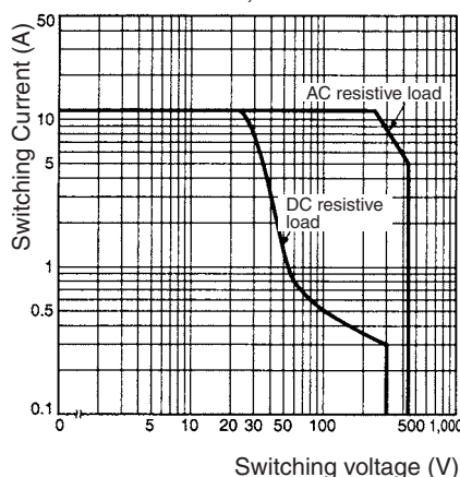
G2RL-1A, G2RL-1
