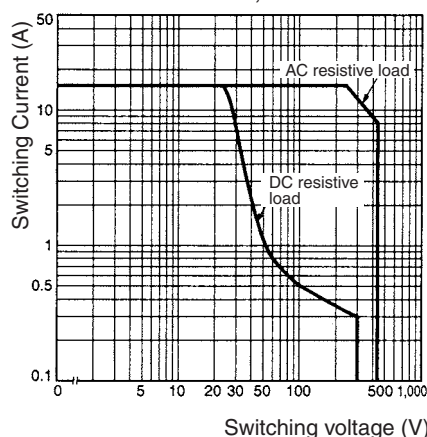
G2RL-1A-E, G2RL-1-E
