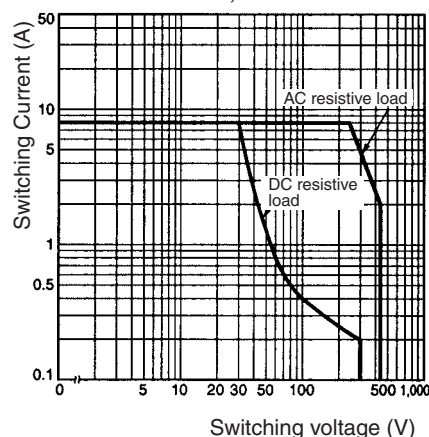
G2RL-2A, G2RL-2
