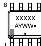
SOIC8, SOIC-8 EP
