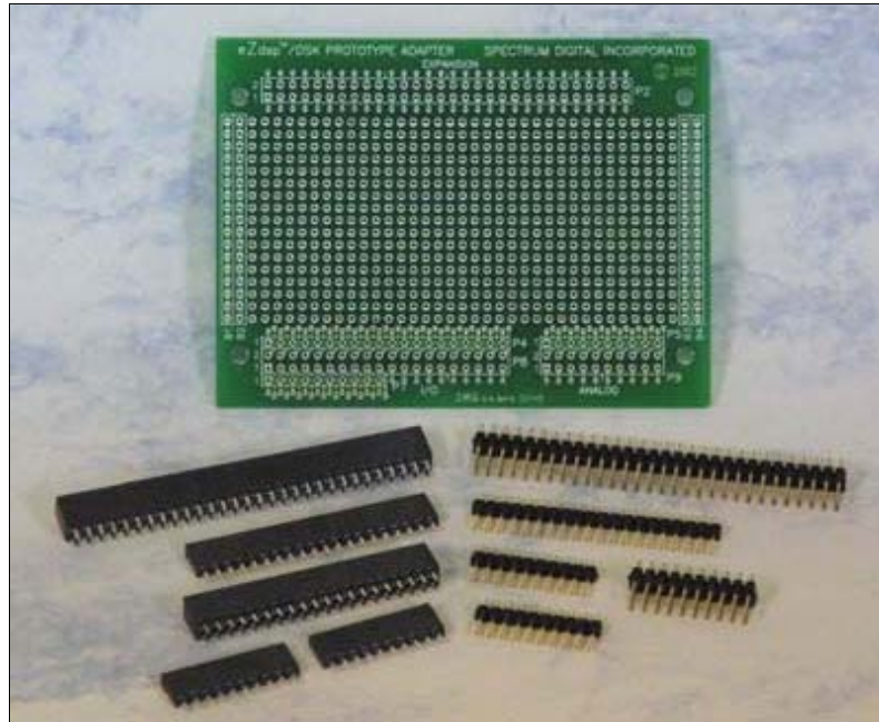
Wire Wrap Prototyping Module for eZdsp
