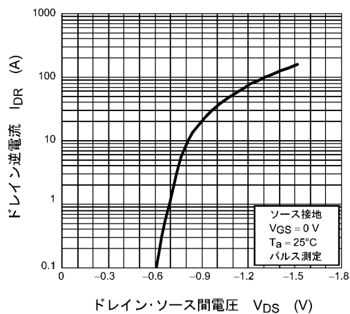
図 8.8 I_{DR} - V_{DS}
