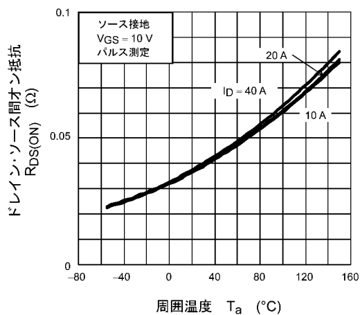
図 8.7 R_{DS(ON)} - T_a
