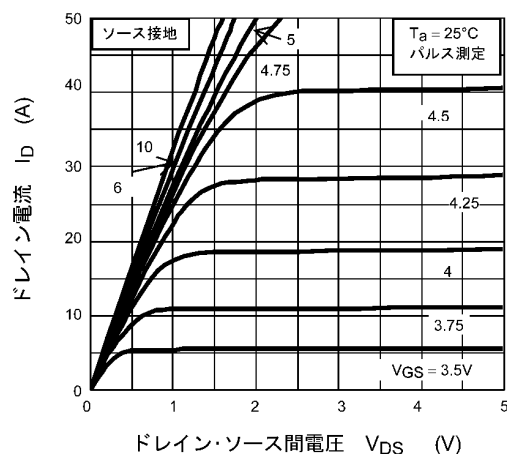
図 8.2 I_D - V_{DS}
