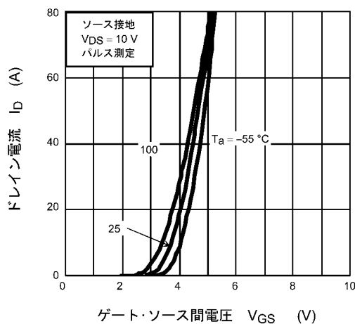
図 8.3 I_D - V_{GS}
