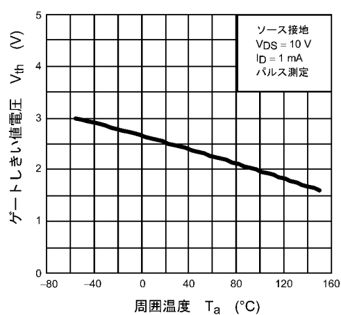
図 8.10 V_{th} - T_a
