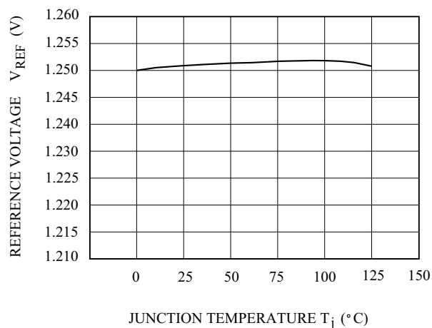
Fig. 4 V_{REF} - T_j
