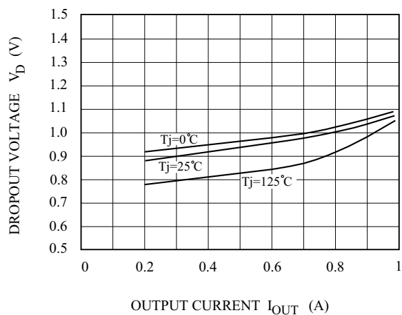
Fig. 3 V_D - I_{OUT}
