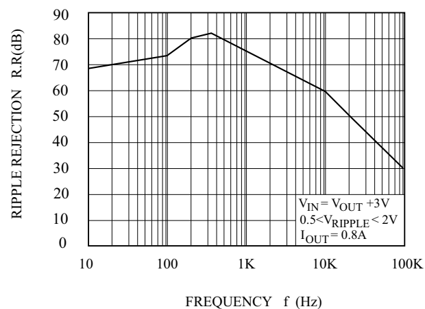
Fig.8 R.R-f
