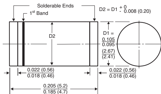
DO-213AB (GL41)
