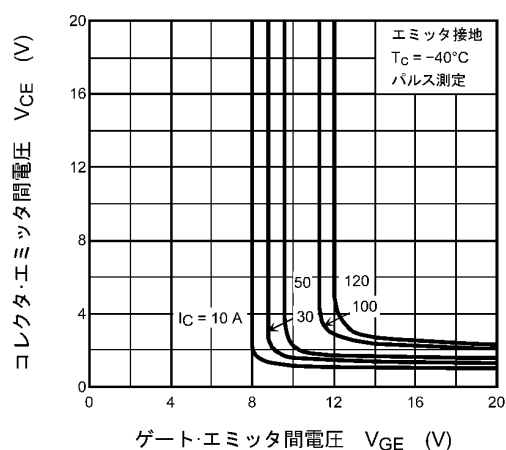
図 8.6 V_{CE} - V_{GE}
