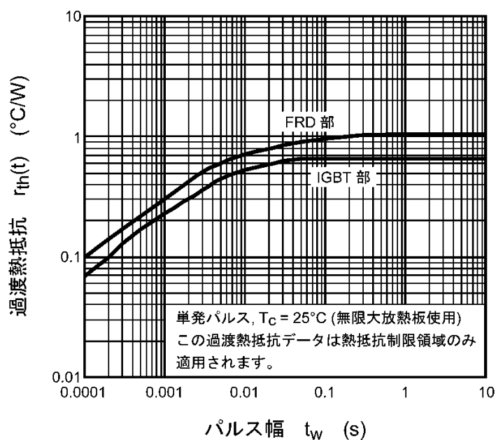
図 8.21 r_{th}(t) - t_w (最大値 (保証値))
