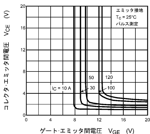
図 8.5 V_{CE} - V_{GE}
