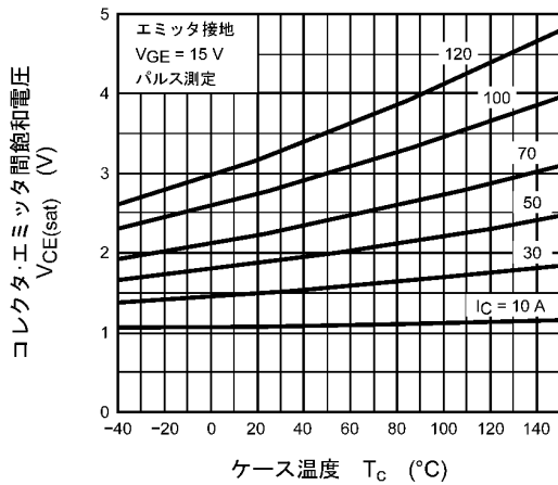
図 8.9 V_{CE(sat)} - T_c
