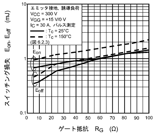
図 8.14 E_{on} , E_{off} - R_G
