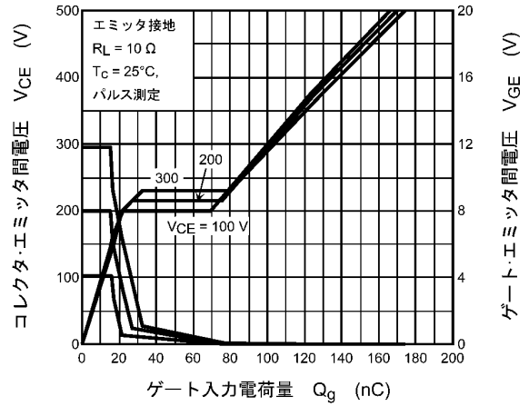
図 8.16 V_{CE} , V_{GE} - Q_g
