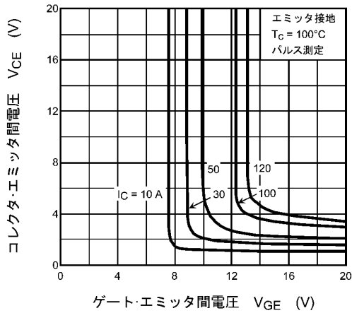
図 8.7 V_{CE} - V_{GE}
